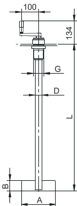
Hand Stirrer
